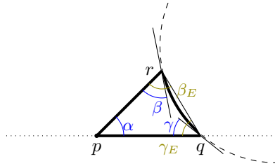
Abb. IV.7.: Ein hyperbolisches Dreieck in \mathbb{D} mit p im Ursprung
