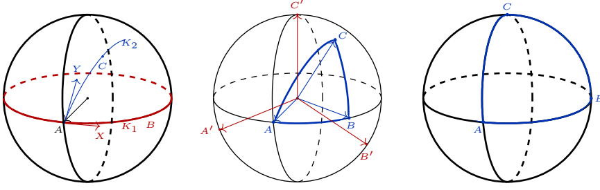
Abb. IV.8.: Links: Definition des Winkels zwischen zwei Großkreisen. Mittig: Das Polardreieck A'B'C' zum Dreieck ABC . Rechts: Ein Dreieck mit drei rechten Winkeln.
