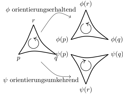
Abb. III.3.: Orientierung von Dreiecken
