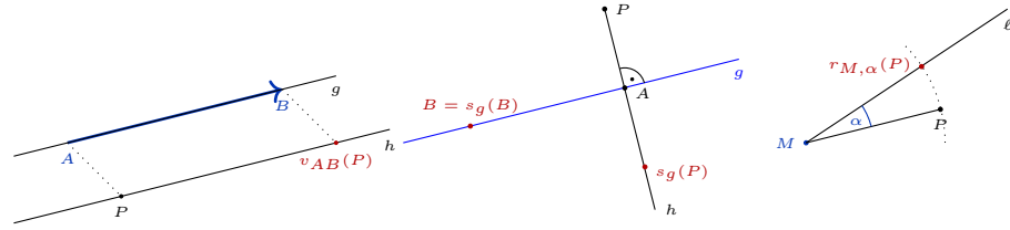
Abb. III.1.: Links: Verschiebung v_{AB} , Mitte: Spiegelung s_g , Rechts: Drehung r_{M,\alpha}
